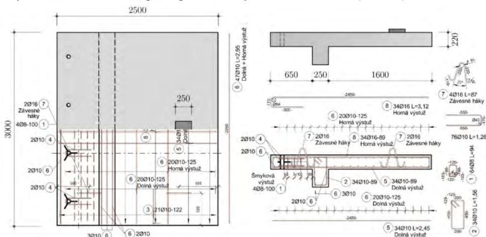
Obr.5.1 Tvar a schéma vyztuženia experimentálnej dosky
