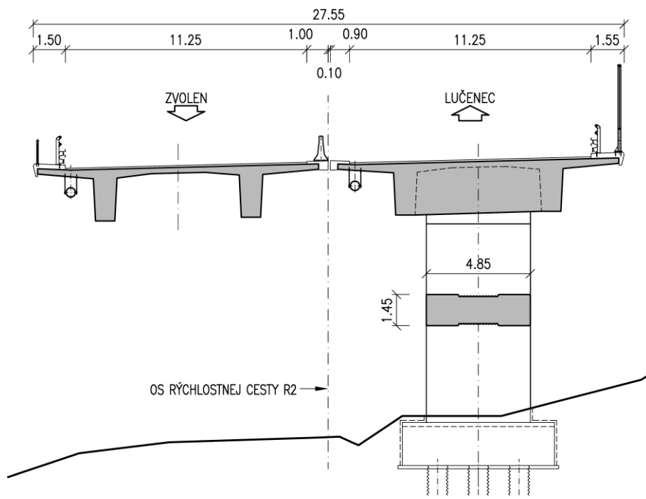
Obr. 5 – 210-00 - Usporiadanie v priečnom smere
