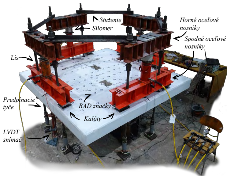
Obr.2.3- Skúšobná zostava
