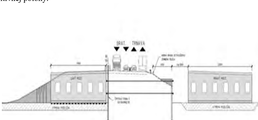
Obrázok č.3 – Jedna z projektovaných fáz výstavby
