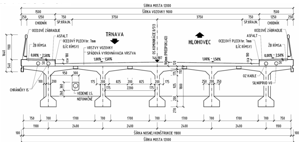
Obr. 2 Priečný rez mostom, nosníková časť, pôvodný stav
