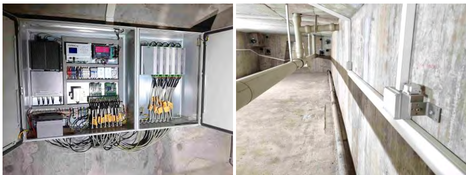
Obr. 7 Kabeláž od snímačov zvedená do meracích skriň a zapojená do PC zostavy
