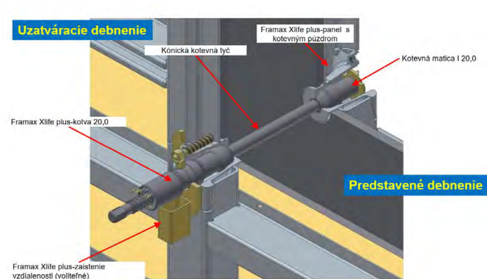
Obr. 2: Riešenie jednostranne ovládateľného kotvenia rámového debnenia Framax Xlife plus
