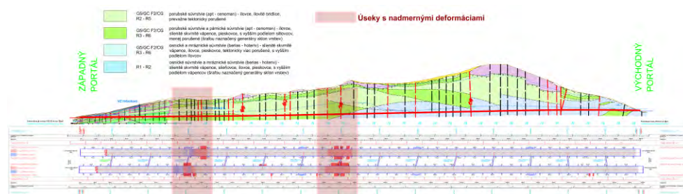
Obr. 1 Inžinierskogeologický profil
