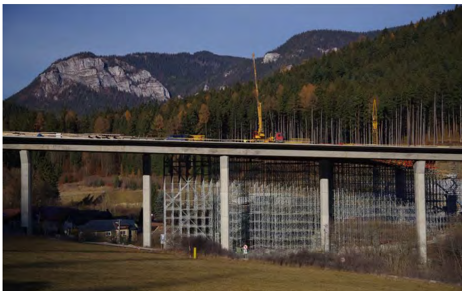
Obr. 8- Postupná betonáž polí ramp
