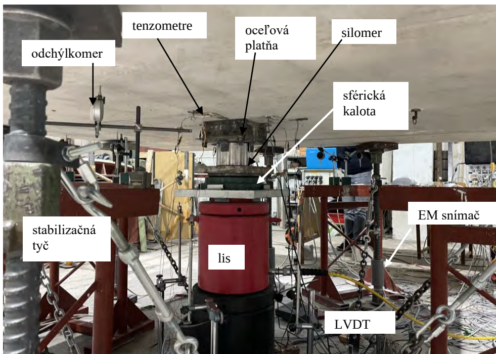
Obr. 4.2 Experimentálna zostava
