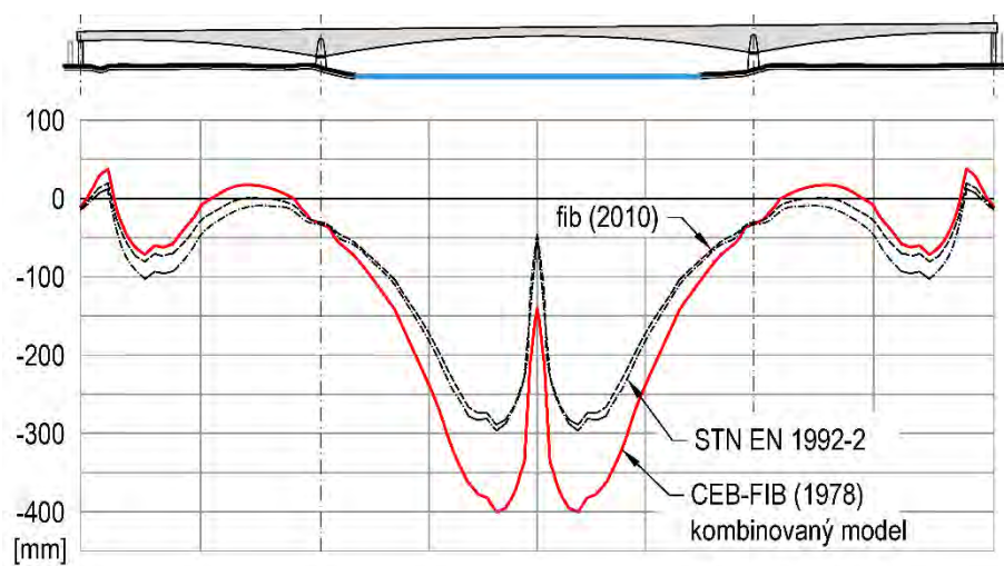
7. Výpočet nadvýšenia
