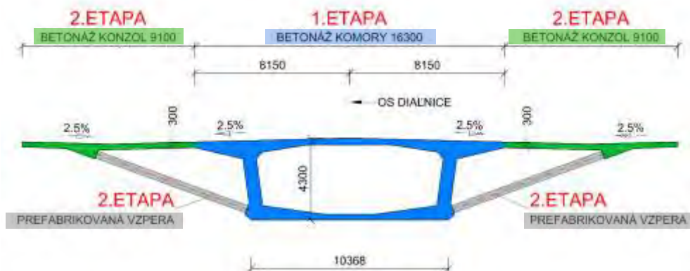
Obr. 2 Charakteristický priečný rez – zhotovenie v dvoch etapách
