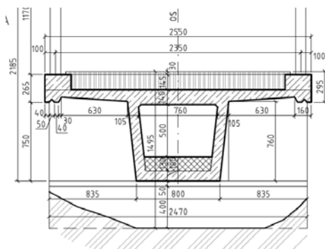
Obr. 1: Schematický priečny rez konštrukciou.
